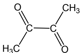
Butane-2,3-dione
