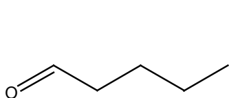
i. pentanal
