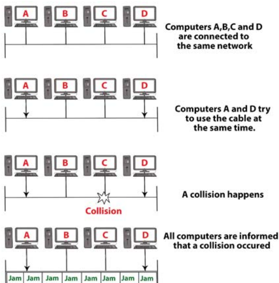
Figure 2.1.: CSMA/CD
